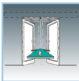
MI 6020/6120 Разблокировочная система для 2 подвижных створок (шириной 1100/1500 мм)
